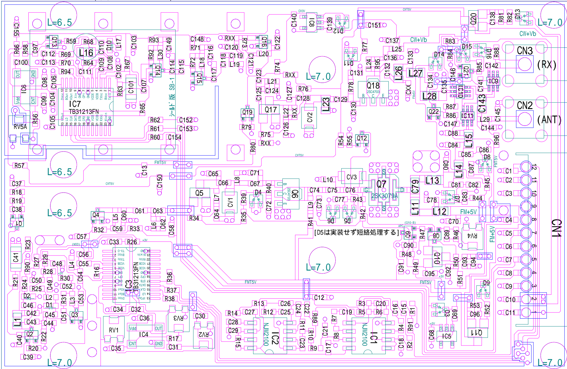
TXE430MFCW-301A送信基板図
