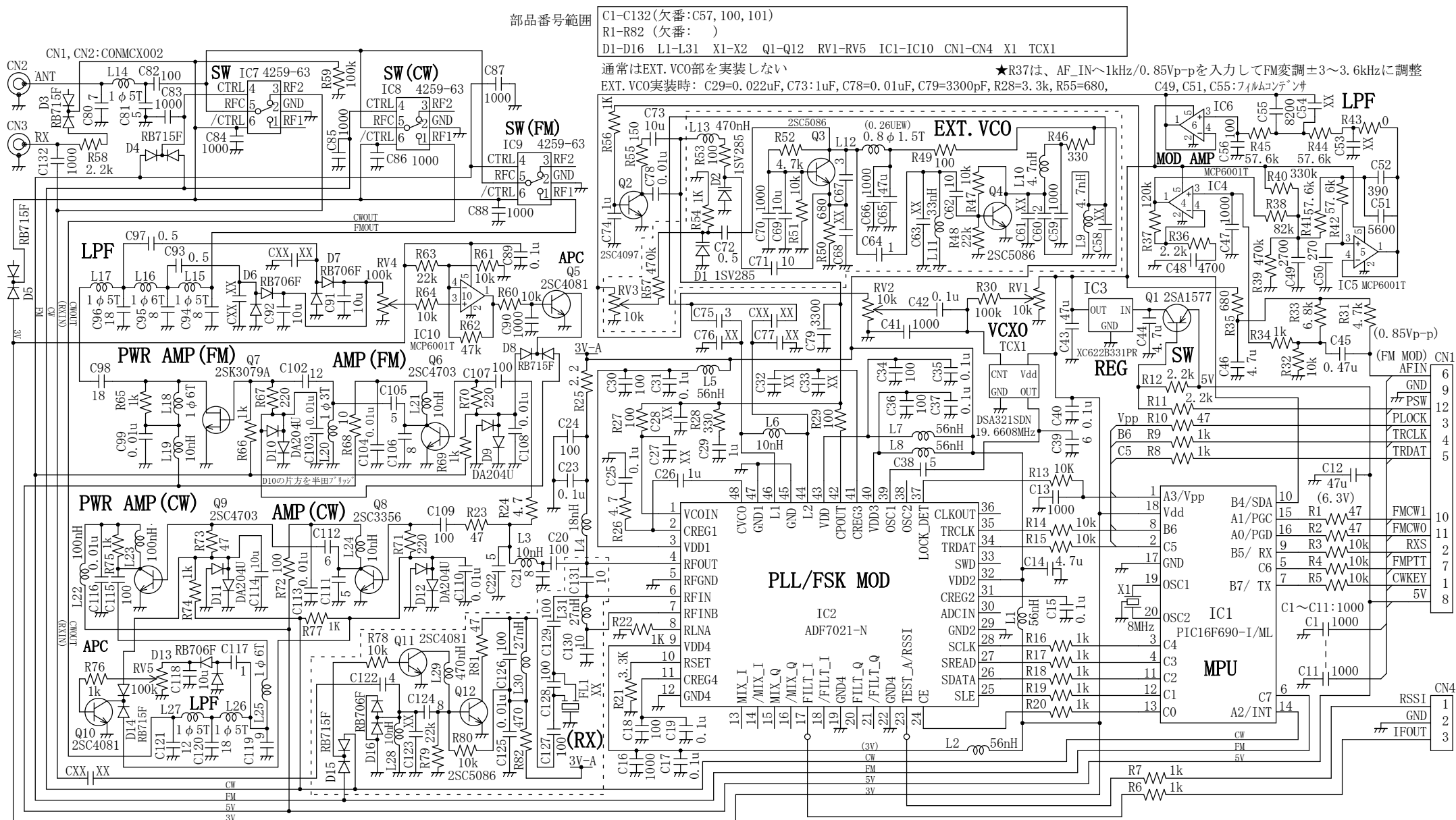
FMCW送信機回路図 TXE430MFMCW-302A
