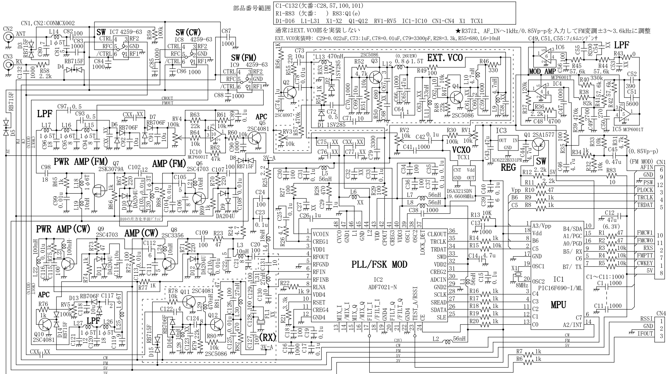
FMCW送信機回路図 TXE430MFCW-302A
