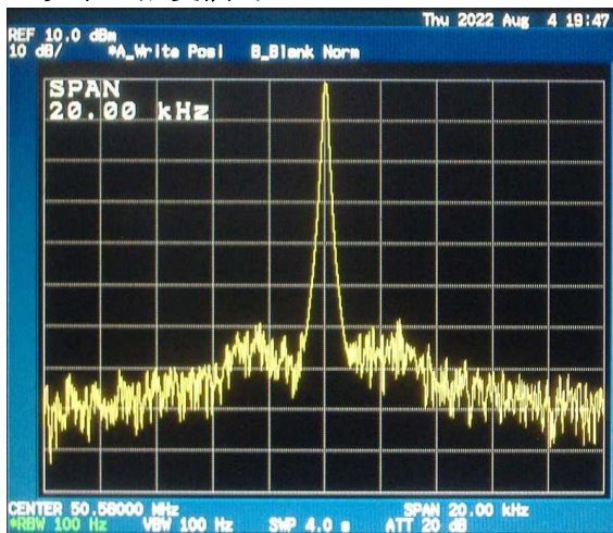
以下は無変調時のスペクトル
