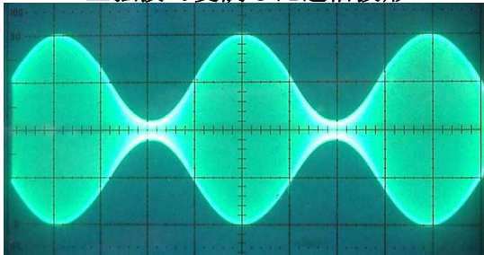
1kHz正弦波で変調した送信波形
