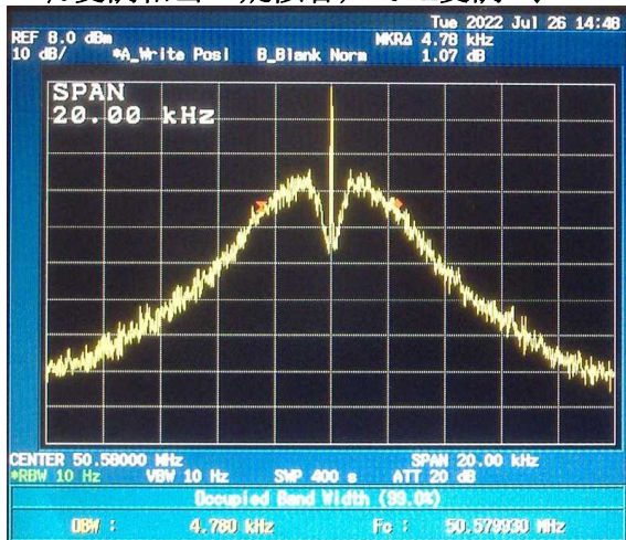
(占有帯域幅：4.78kHz)
